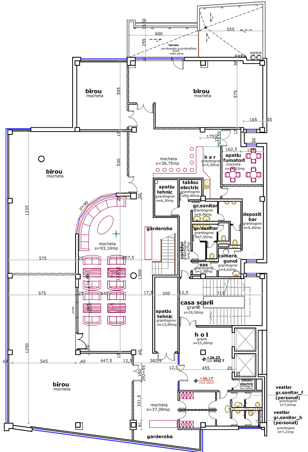
plan etaj 7 _ scara 1:200
