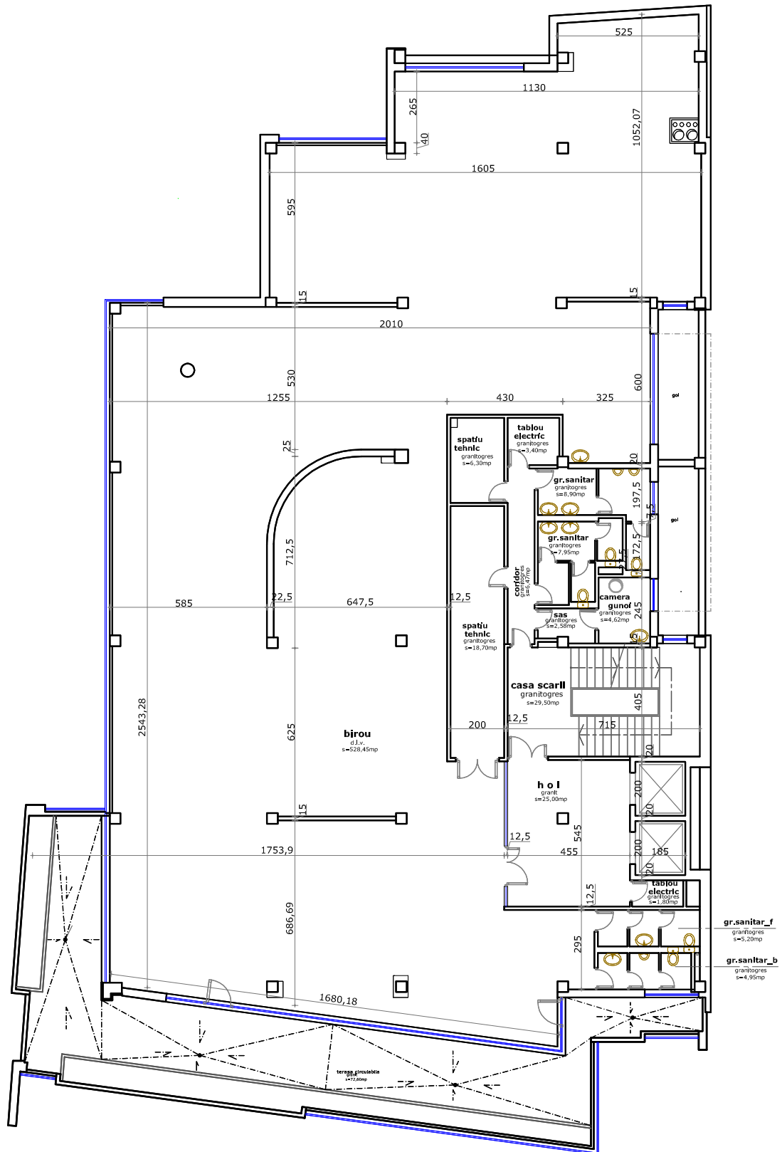
plan etaj 6 _ scara 1:200
