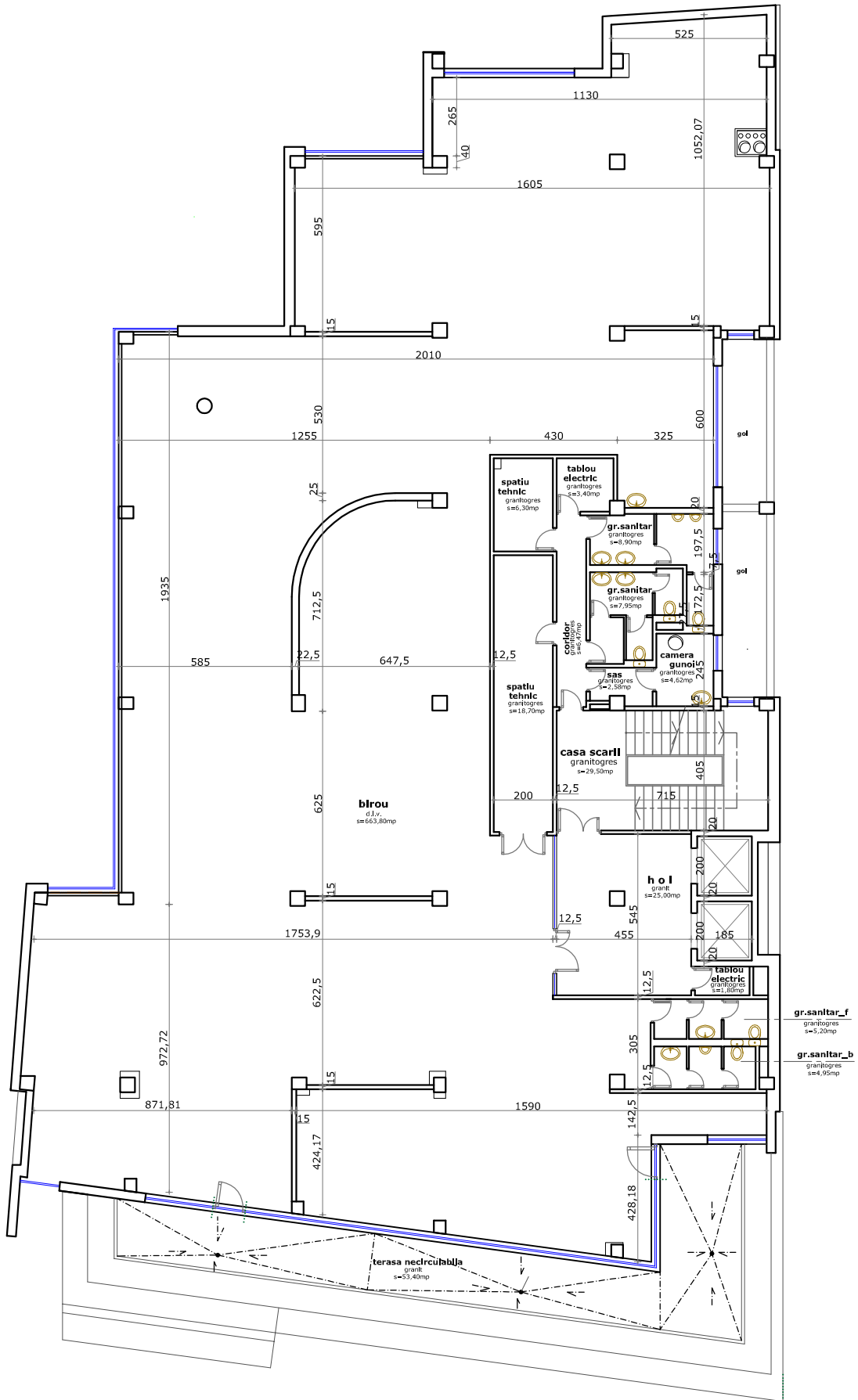
plan etaj 4_ scara 1:200
